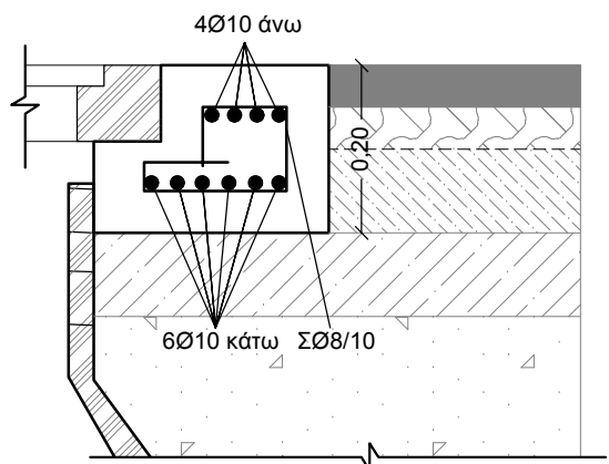
ΛΕΠΤΟΜΕΡΕΙΑ Λ1 - ΟΠΛΙΣΜΟΣ ΣΤΗΝ ΤΟΜΗ Α-Α' ΚΛΙΜΑΚΑ 1:10
