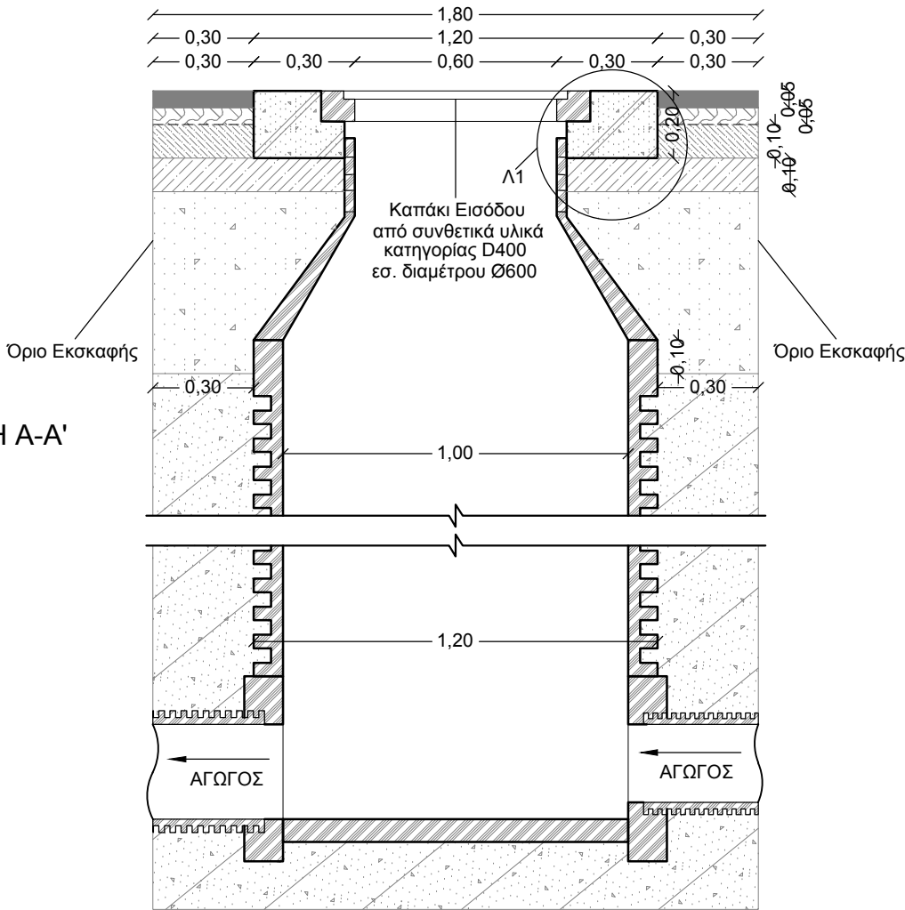
ΤΟΜΗ Α-Α' ΚΛΙΜΑΚΑ 1:20
