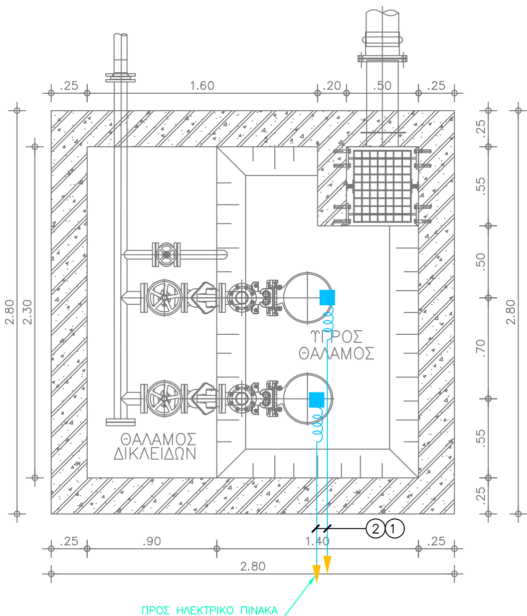
ΟΡΙΖΟΝΤΙΑ ΤΟΜΗ
