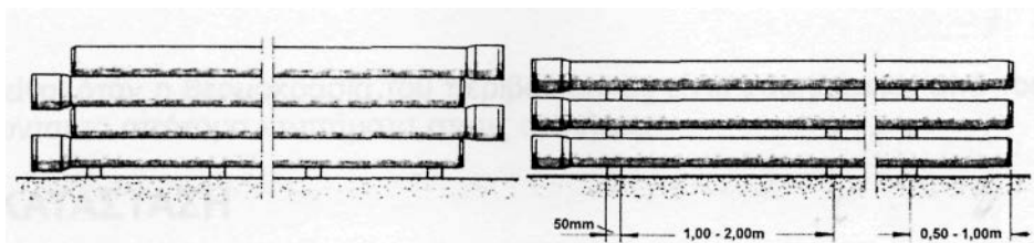
Σχήμα 3.11: Τοποθέτηση των σωλήνων.
