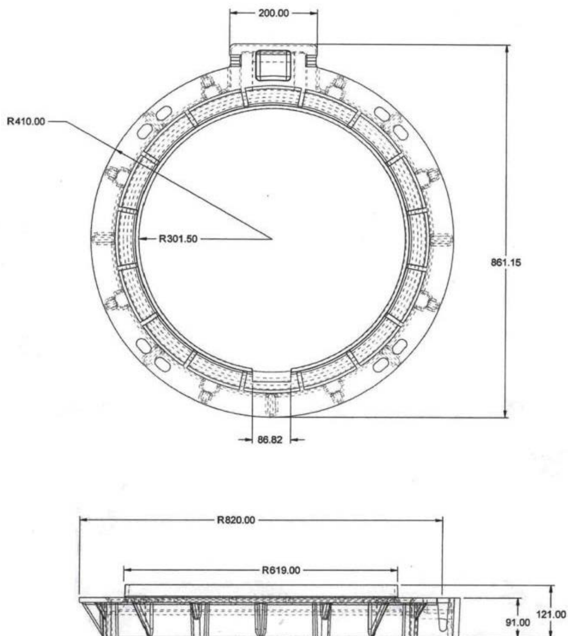
Σχήμα 3.5: Κάλυμμα φρεατίου από συνθετικό υλικό
