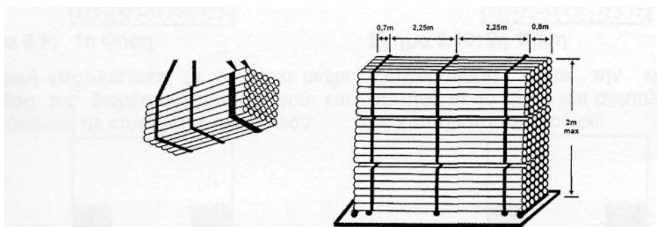
Σχήμα 3.12: Αποθήκευση των ευθέων σωλήνων.
