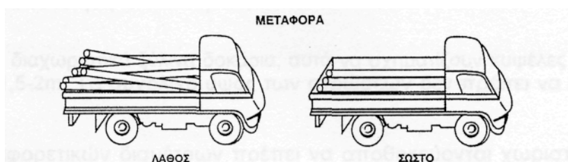
Σχήμα 3.9: Σωστός και ανορθόδοξος τρόπος μεταφοράς σωλήνων.
