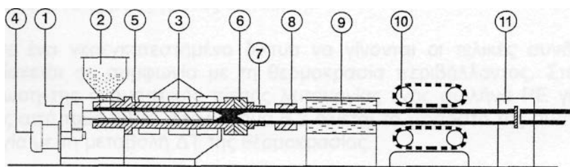
Σχήμα 3.6: Παραγωγή των σωλήνων HDPE με τη μέθοδο της εξέλασης.
