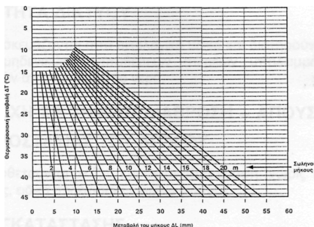
Σχήμα 3.7: Ποσοστό της συστολοδιαστολής σε αναλογία με τη μεταβολή της θερμοκρασίας.
